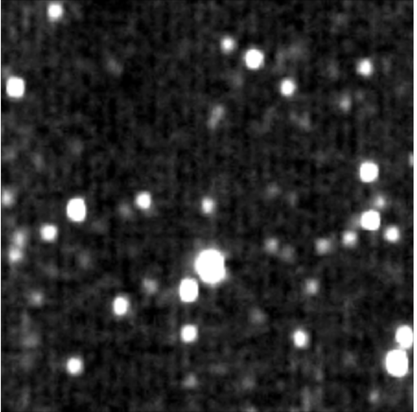
هذه الصورة التي التقطتها مركبة نيو هورايزنز للجرم JR1 1994 الموجود في حزام كايبر، هي أقرب الصور التي تم التقاطها على الإطلاق. المصدر: NASA/JHUAPL/SwRI
